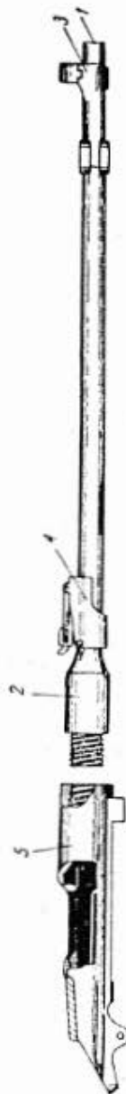
Rys. 144. Lufa z komorą nabojową i zamkową: 1 — przewód gwintowany; 2 — komora nabojowa; 3 — podstawa muszki; 4 — podstawa celownika; 5 — komora zamkowa
