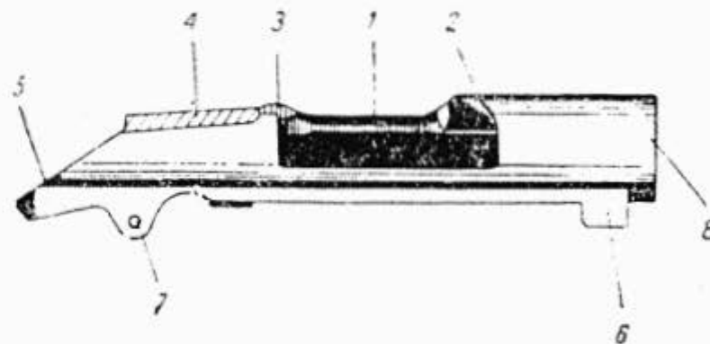
Rys. 146. Komora zamkowa: 1 — górny wąż nabojowy; 2 — skos; 3 — wkład; 4 — górne wodzidło; 5 — ogon; 6 — czop oporowy; 7 — ucho; 8 — gwint
